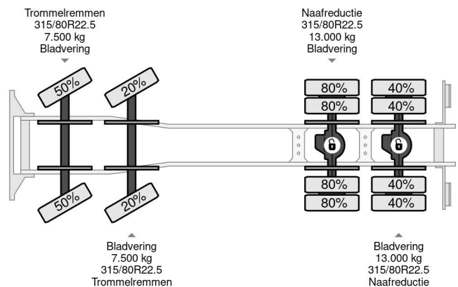
MAN 35 .403DF 8x4 MEILLER KIPPER (EURO2 / ZF16 MA... Referentienummer: SN 60428120
