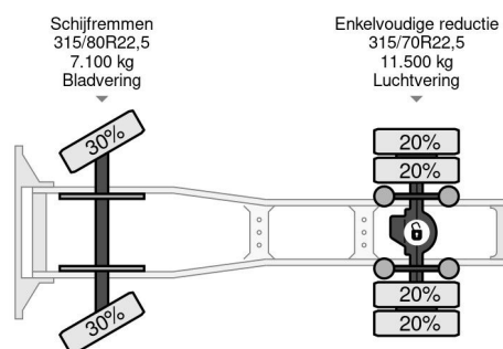
Renault Magnum 440 E-TECH (EURO 3 / ZF16 MANUA... 4x2
