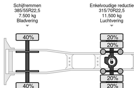
Scania R164-580 V8 TOPLINE COLLECTORS ITEM!! / ... 4x2 Referentienummer: SN 59259678
